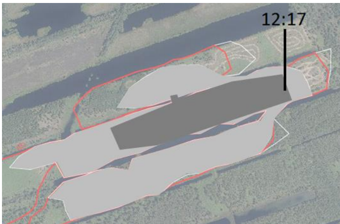
Afbeelding 5.16: Vergelijking van het daadwerkelijke brandverloop (donkergrijs) en het brandverloop volgens het model
