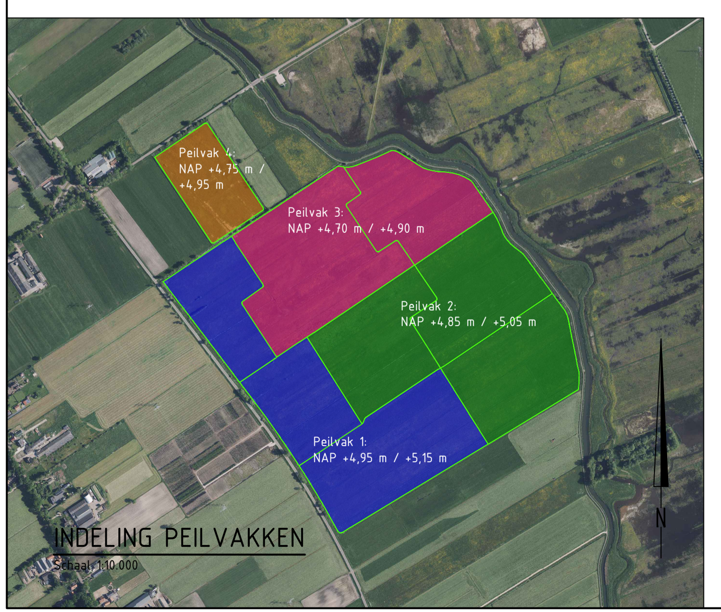
SITUATIE Schaal 1:2.000
