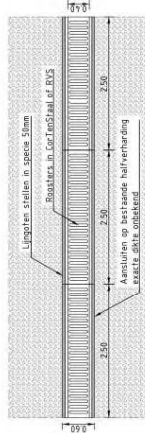
Detail: lijngoot (ACO Exodrain o.g.) Schaal 1:50
