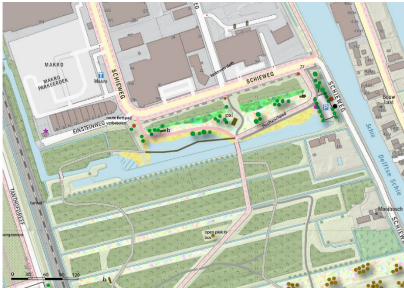
Afbeelding: schetsontwerp met watercompensatie en ontbrekende schakel fietspad en vlonderpad (uit bijlage 1 schetsontwerp).
