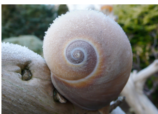
Slakkenhuis met 'poederlaagje' van ijskristallen
